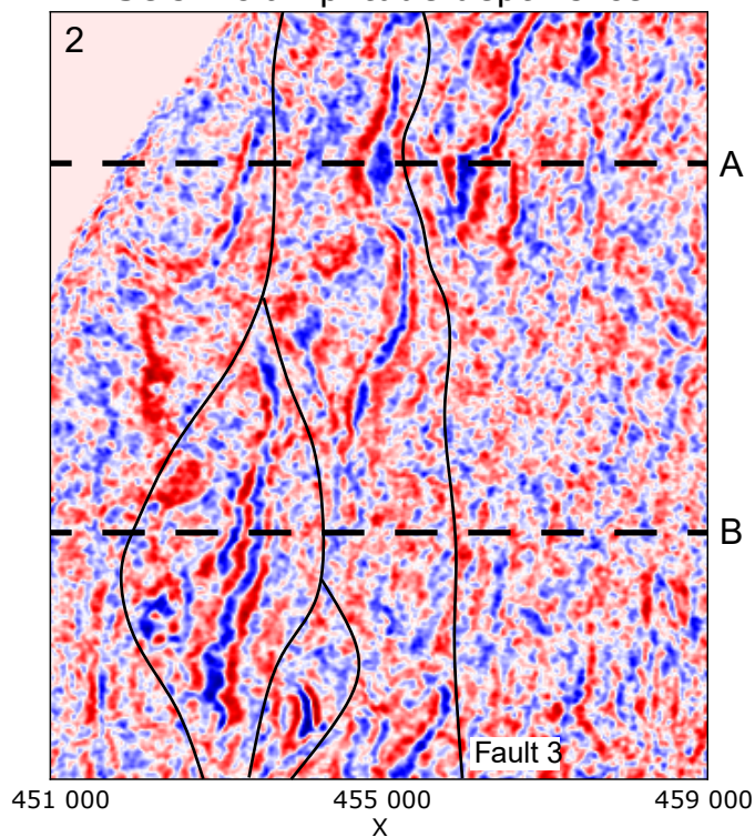
Seismic amplitude depth slice
