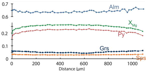
Nordmannvik migmatite
