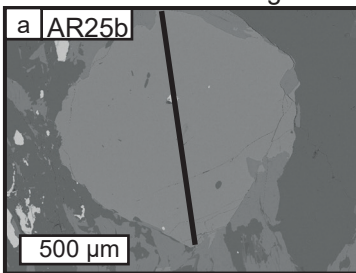
Nordmannvik mylonite
