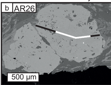
Nordmannvik mylonite
