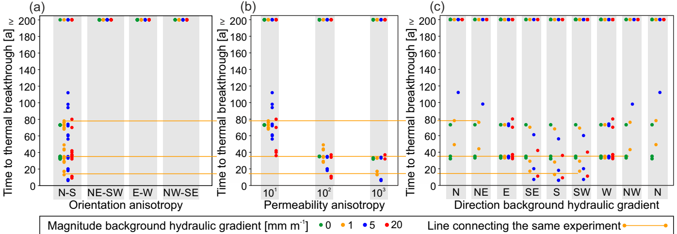
(d) Permeability anisotropy = 10 2 E-W oriented
