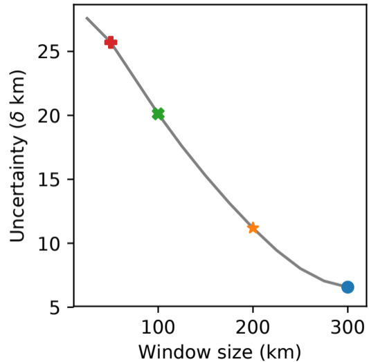
(c) Posterior uncertainty
