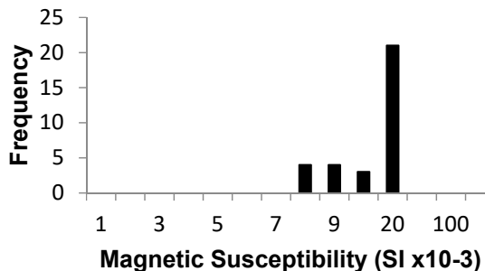
Goodin Inlier n=33
