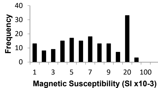
Juderina Formation n=164
