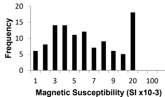
Yarlarweelor GC n=110
