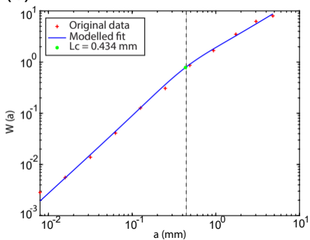
(b) MONTE SUBASIO Scaglia Bianca Fm.
