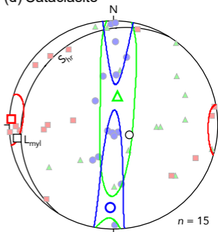
(d) Cataclasite
