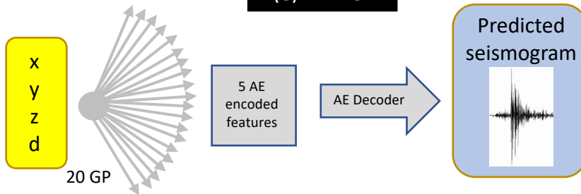
(e) AE + GP
