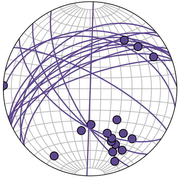
Vein (Quartz, Aplite, Pegmatite)
