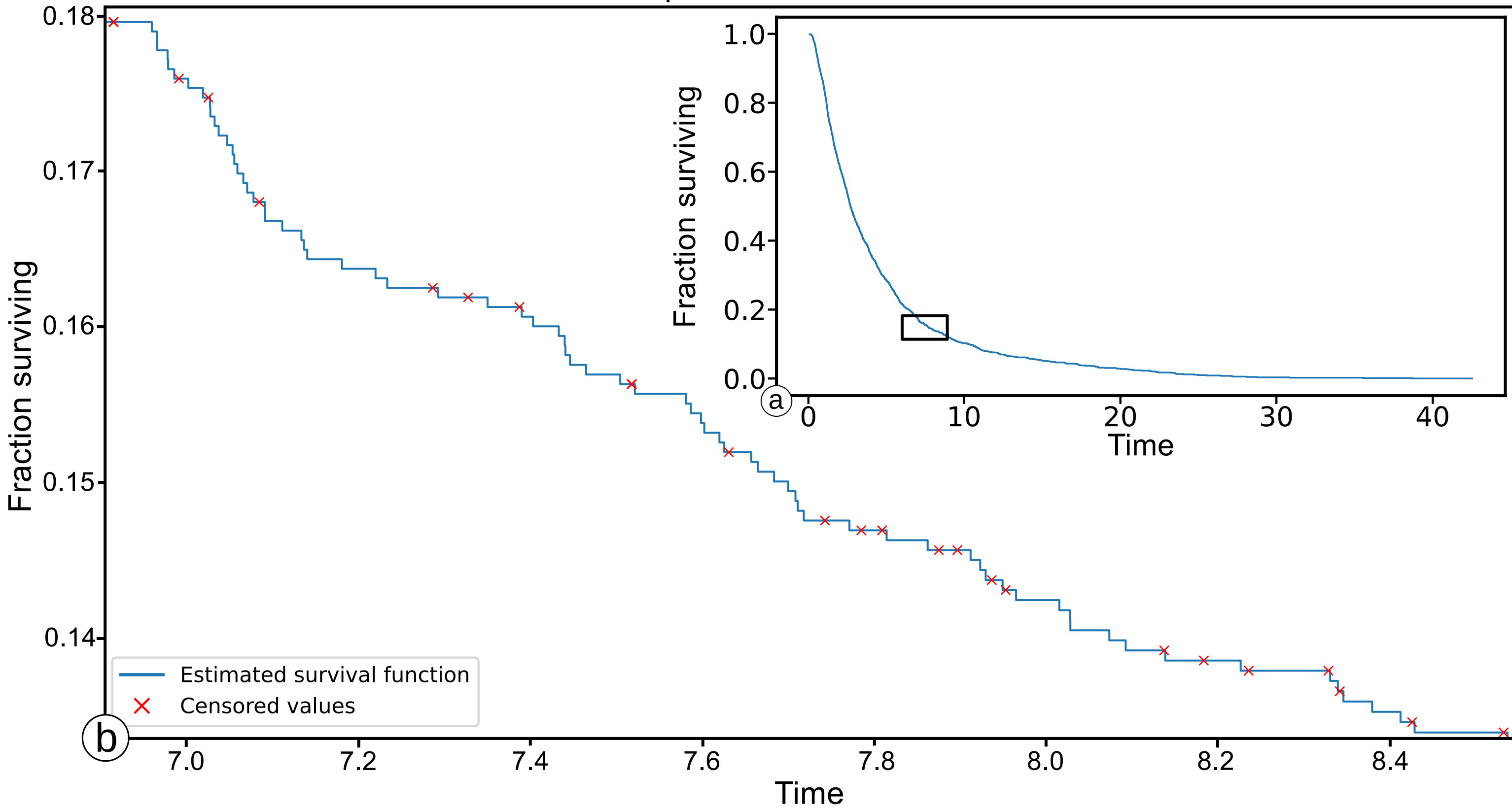
Kaplan-Meier estimator
