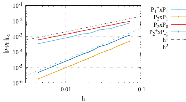
(d) unstructured mesh
