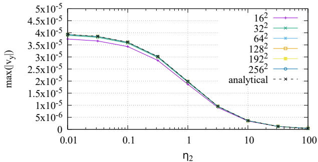
Q_2 \times Q_1
