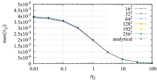
P_2^+ \times P_{-1}
