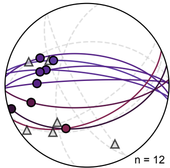
(d) Subdomain D Gastern
