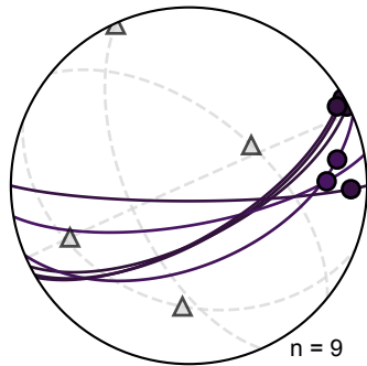
(a) Subdomain A Aiguilles Rouges
