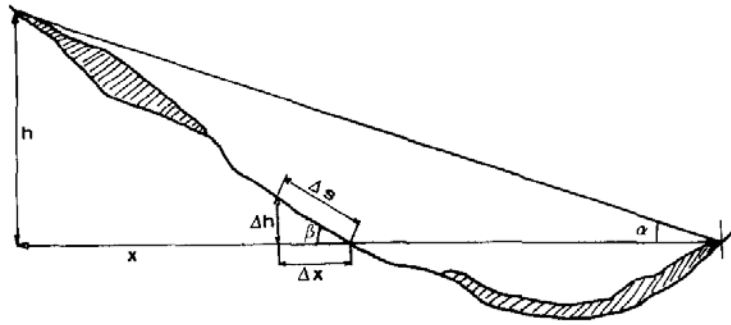
Fig. 1. Geometry of a landslide Geometrie eines Bergsturzes Géometrie d'un éboulement
