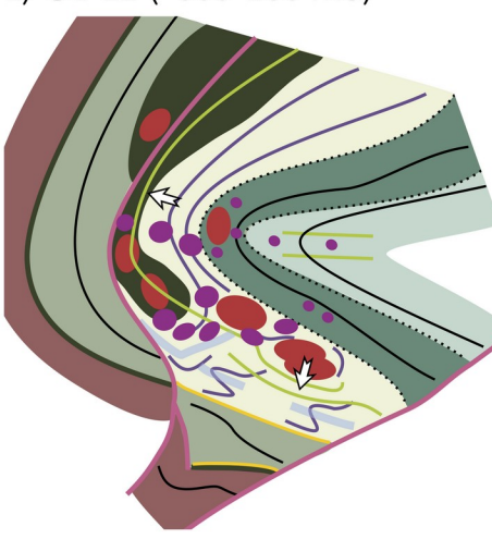
E) C4-E2 (~300-280 Ma)
