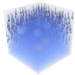
(d) 8 inclusions, \lambda_1/\lambda_0 = 10^4
